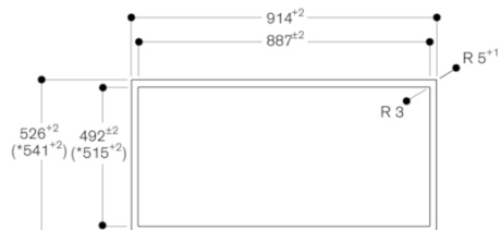
Вид сверху
