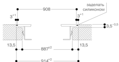
Продольный разрез
