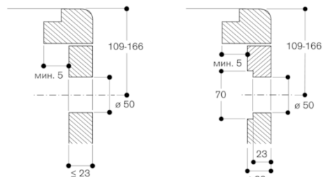
Монтаж регулятора, установка на одном уровне со столешницей
