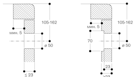
Монтаж регулятора, монтаж на поверхности
